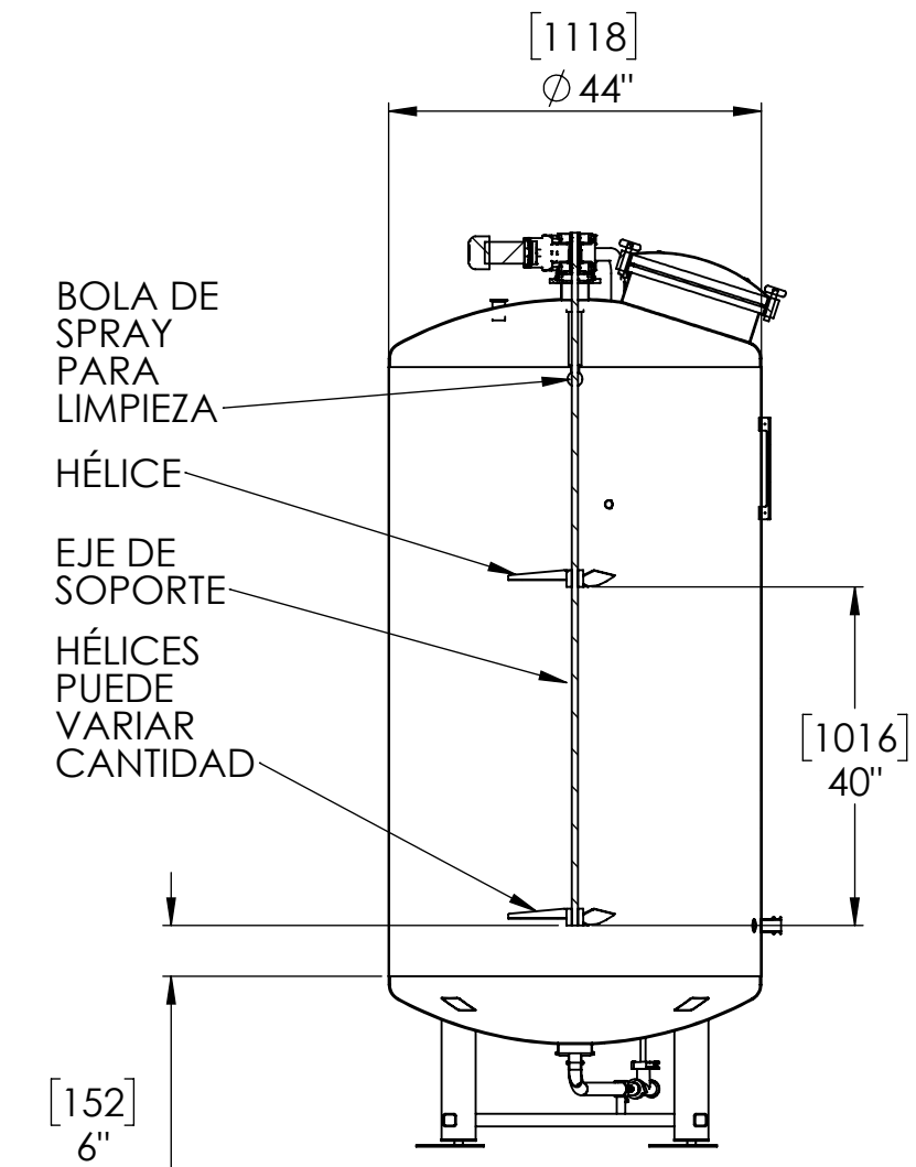
SECCIÓN A-A
